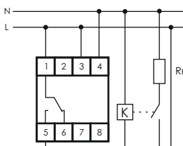
Rn - подключаемая нагрузка K - контактор
